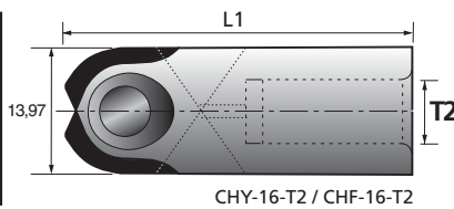
CHY-16-T2 / CHF-16-T2
